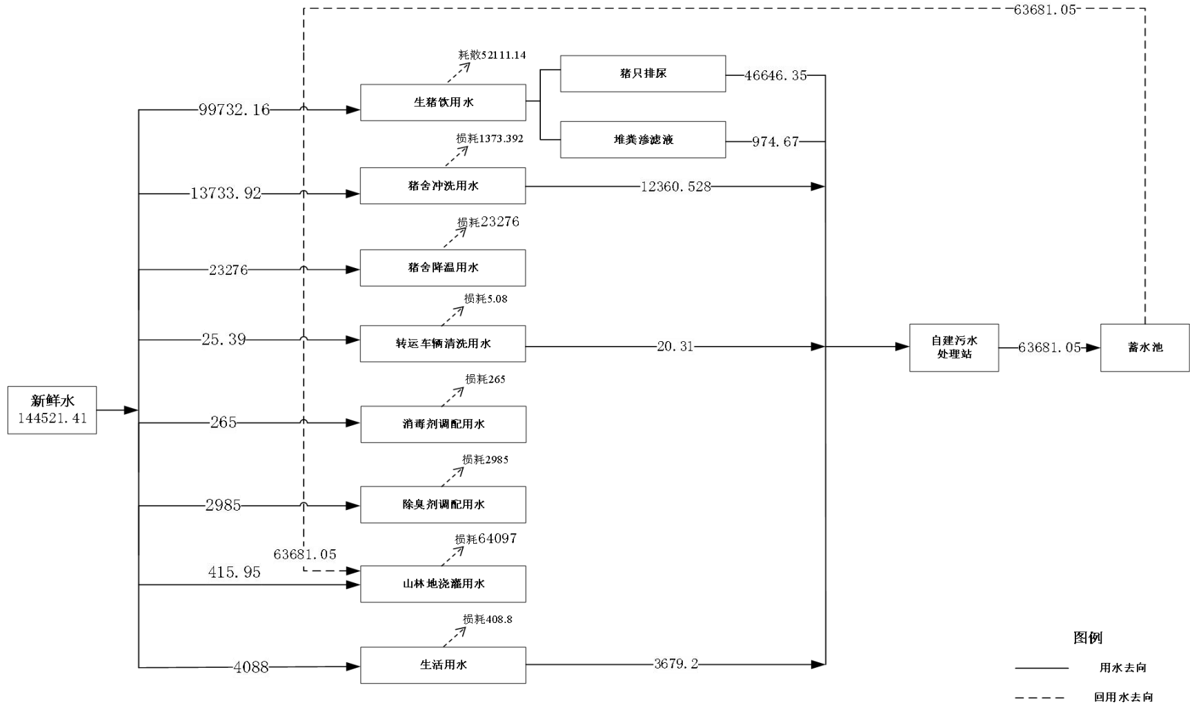
图 3.3-1 项目给排水平衡图（单位：t/a）
