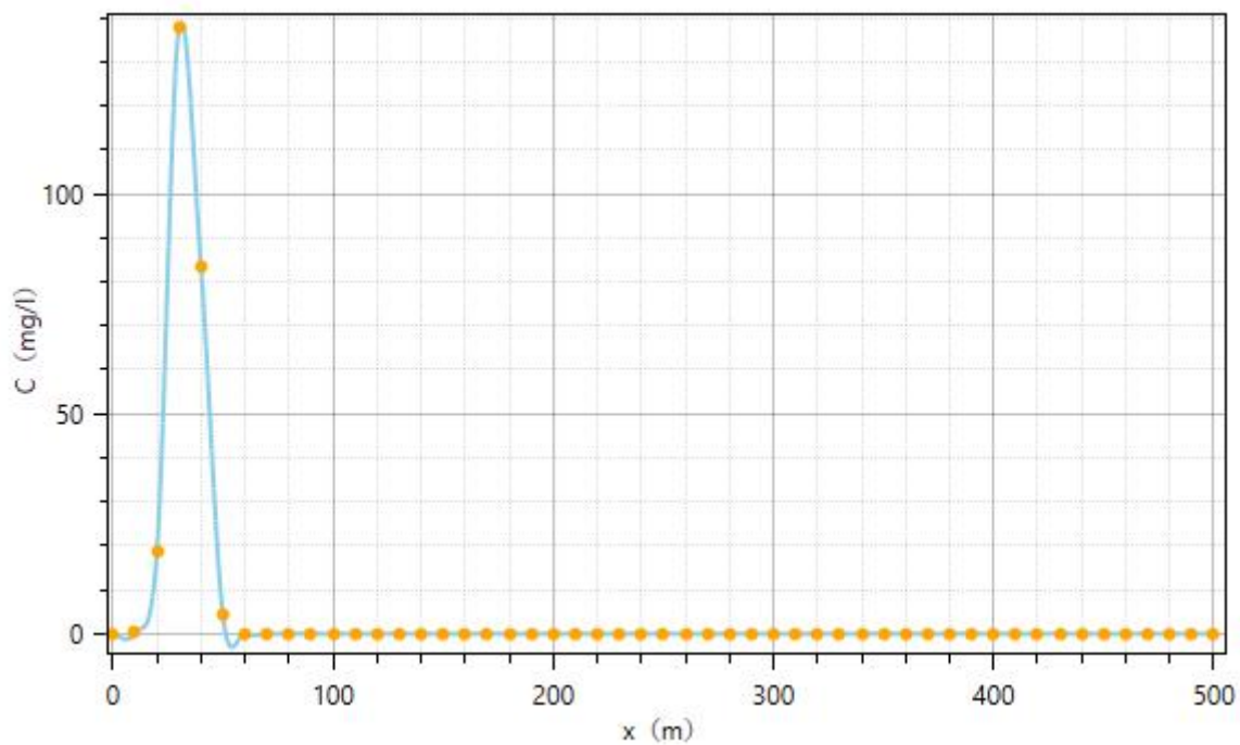
图 5.6-6 污水处理设施污水池及污水管道破裂 100 天氨氮不同距离浓度预测曲线
