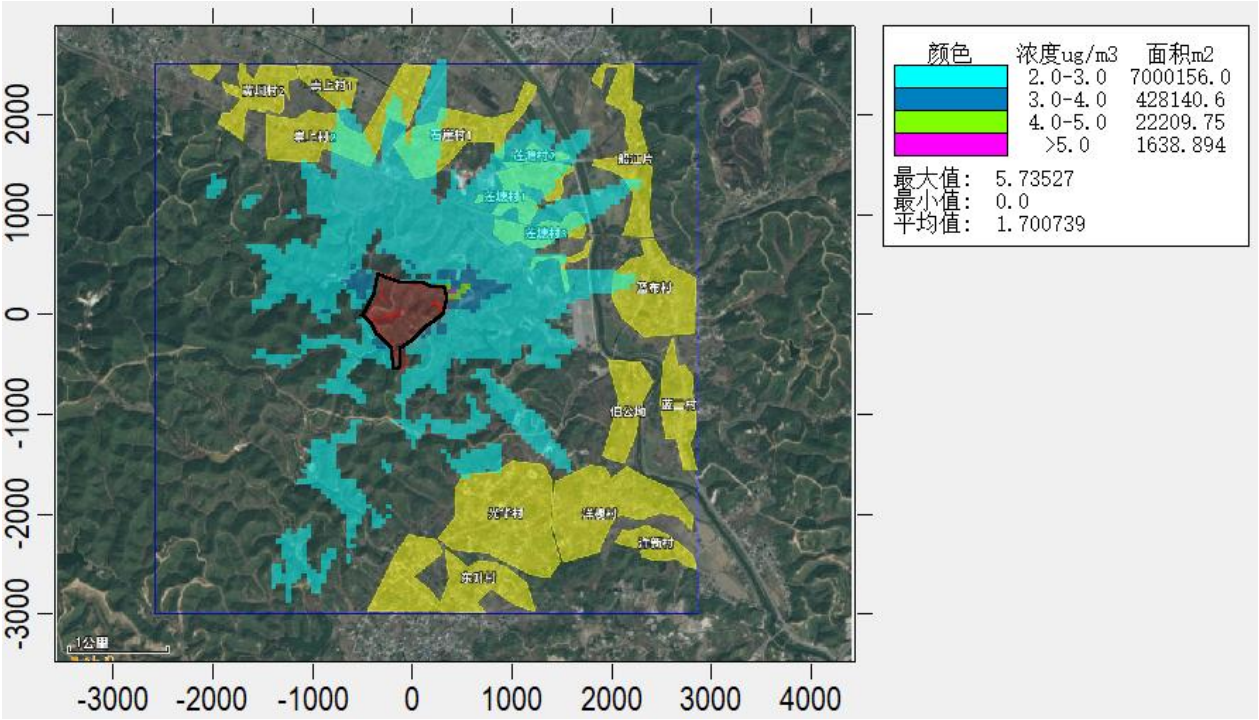
图 5.2-17 叠加后硫化氢小时贡献质量浓度预测等值线图 ( \mu\text{g}/\text{m}^3 )
