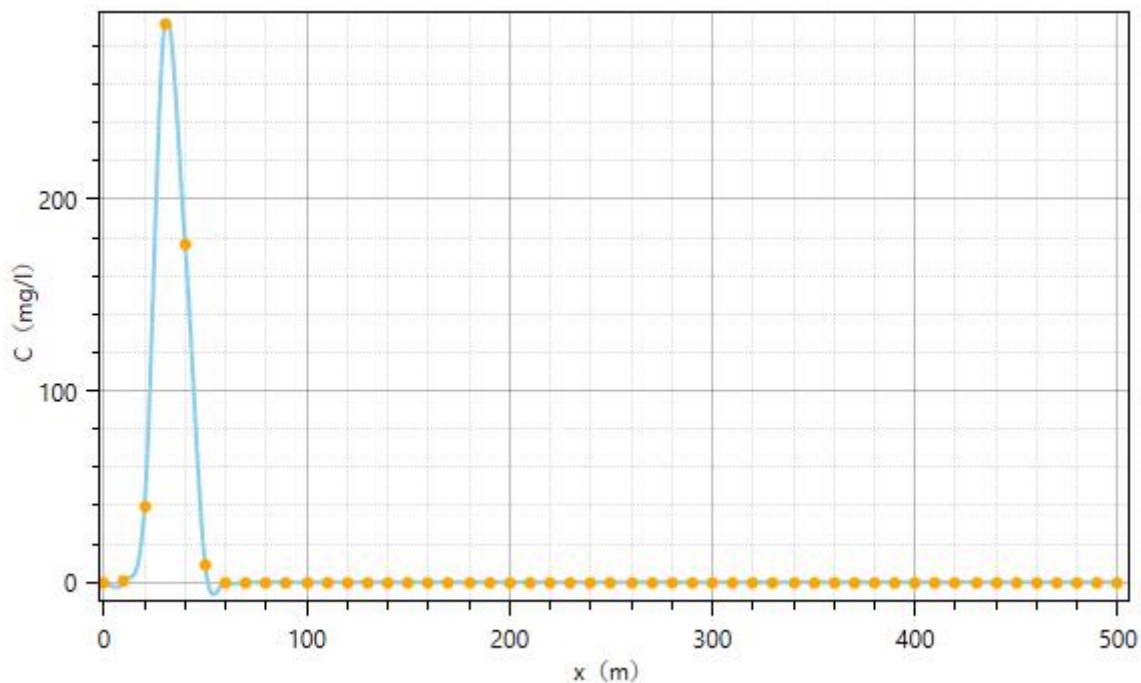
图 5.6-4 污水处理设施污水池及污水管道破裂 100 天 COD 不同距离浓度预测曲线
