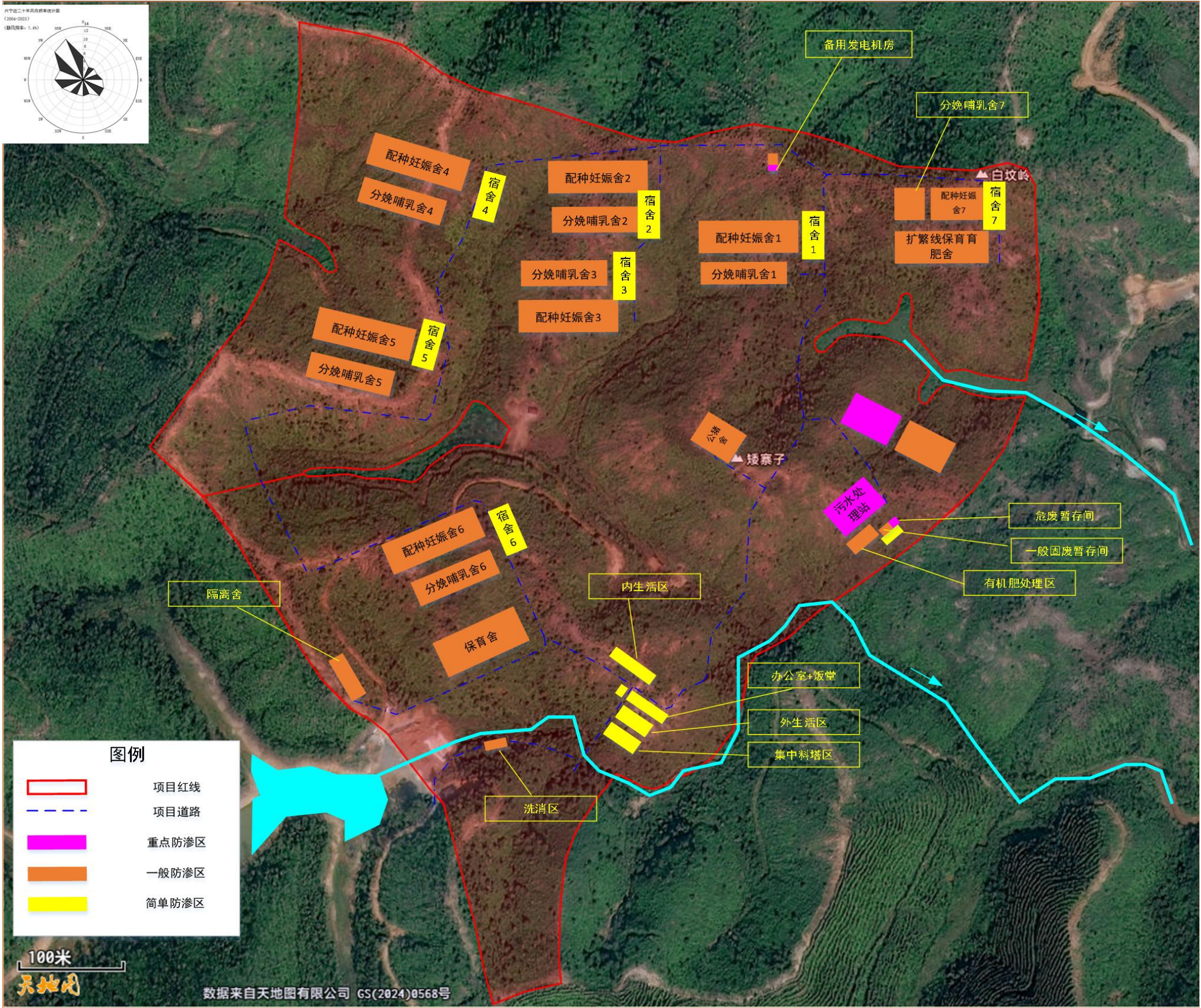
图 5.6-6 本项目分区防渗图
