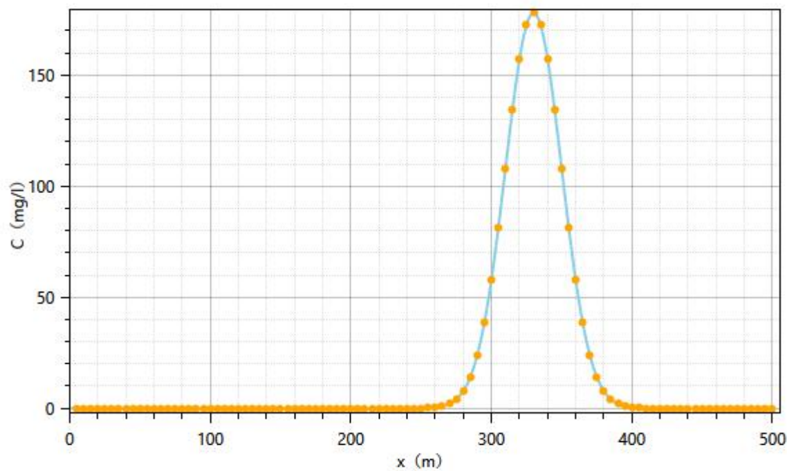
图 5.6-3 储罐破损渗漏 1000 天石油类污染物不同距离浓度预测曲线
