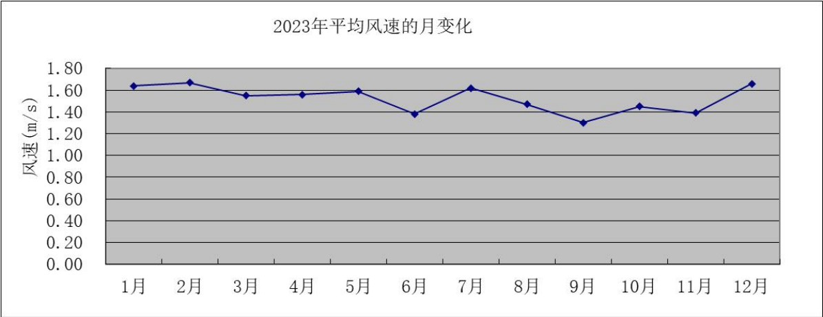
图 5.2-5 兴宁市 2023 年年平均风速月变化曲线图
