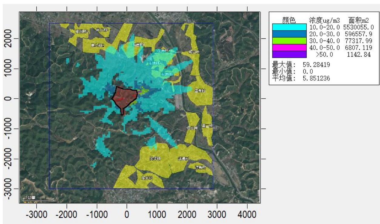
图 5.2-12 氨正常排放小时贡献质量浓度预测等值线图 ( \mu\text{g}/\text{m}^3 )
