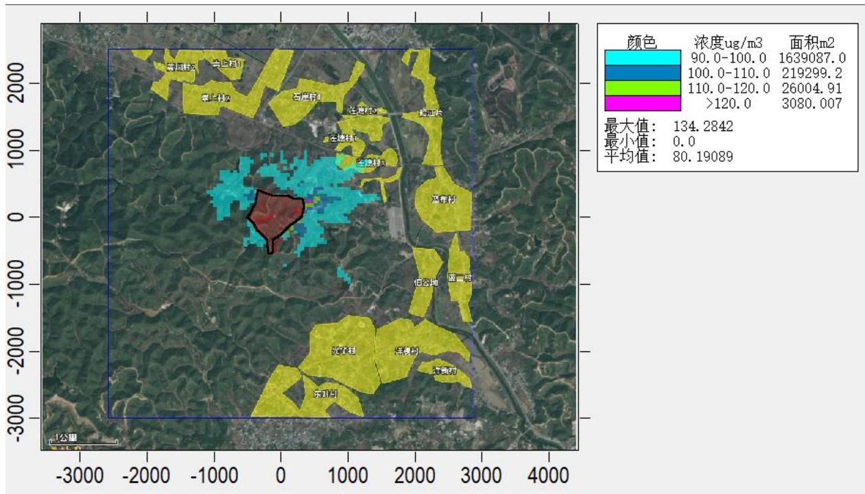
图 5.2-13 叠加后氨小时质量浓度预测等值线图（ \mu\text{g}/\text{m}^3 ）
