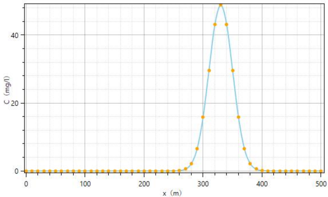
图 5.6-7 污水处理设施污水池及污水管道破裂 1000 天氨氮不同距离浓度预测曲线
