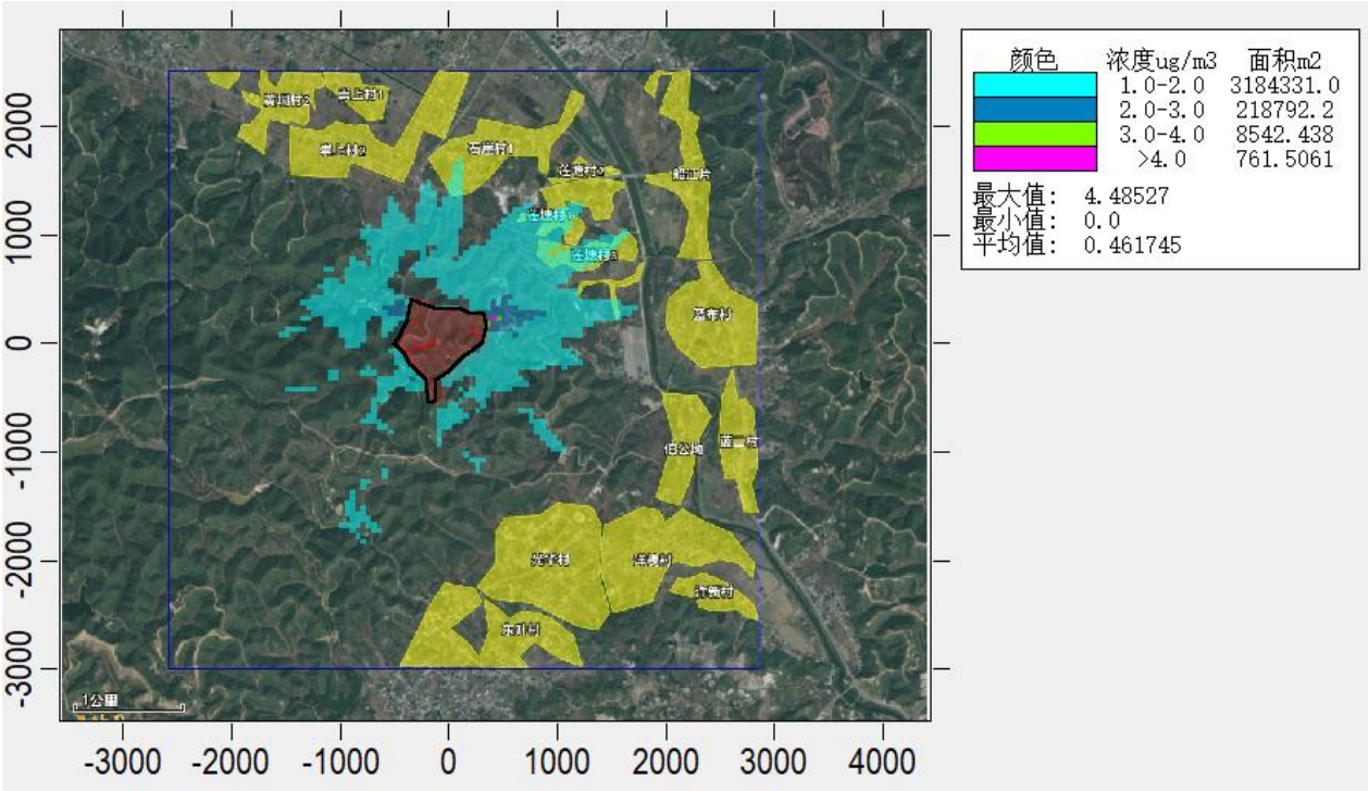
图 5.2-16 硫化氢正常排放小时贡献质量浓度预测等值线图 ( \mu\text{g}/\text{m}^3 )
