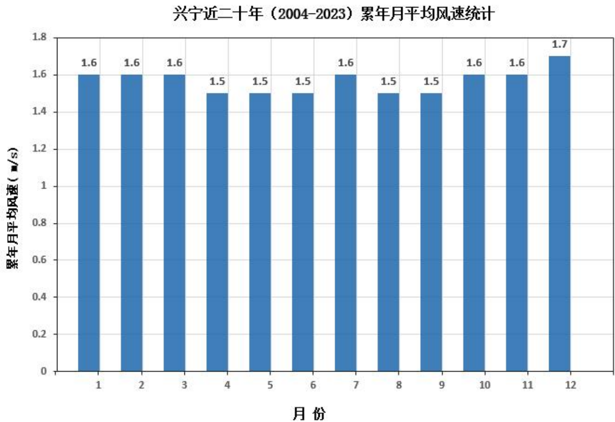
图 5.2-2 兴宁市 2004~2023 年累年月平均风速变化曲线图
