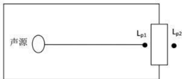
图 5.4-1 室内声源等效为室外声源示意图
