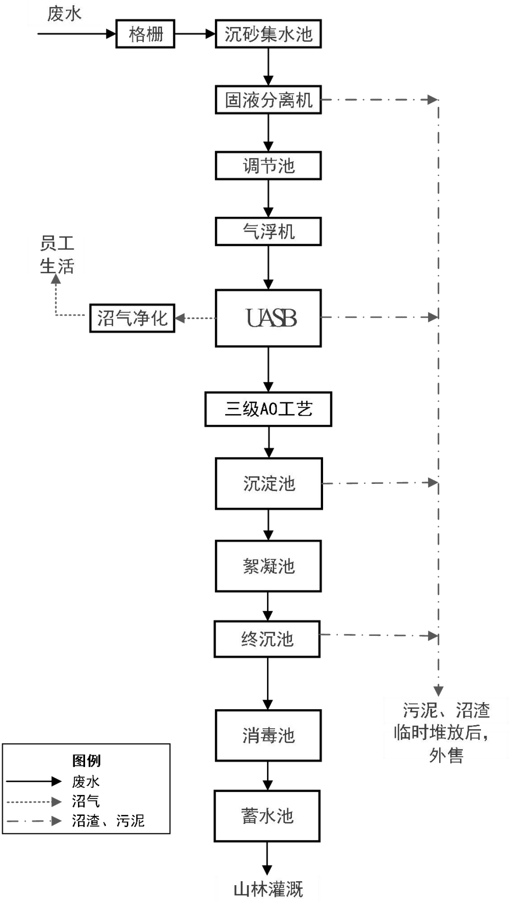
图 7.2-1 项目废水处理工艺流程图
