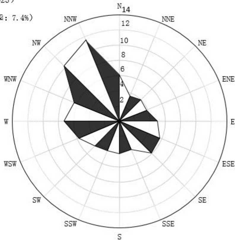
图 5.2-3 兴宁市近 20 年风向频率玫瑰图（统计年限：2004～2023 年）
