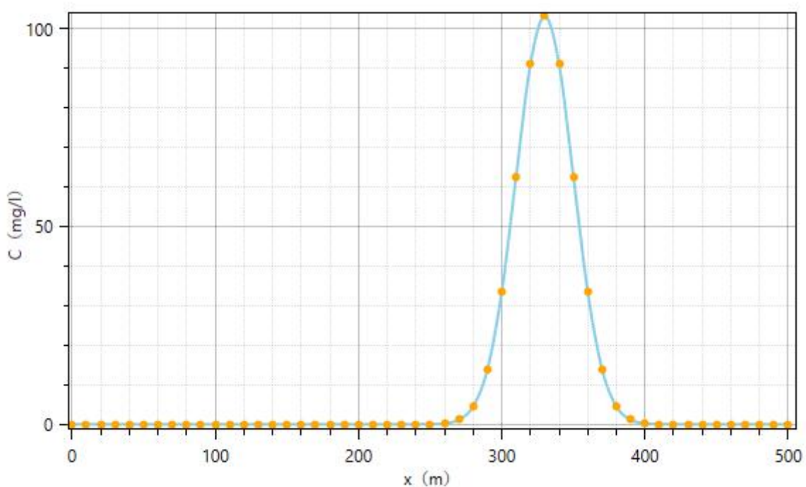
图 5.6-5 污水处理设施污水池及污水管道破裂 1000 天 COD 不同距离浓度预测曲线
