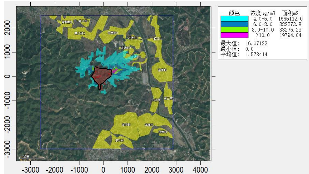
图 5.2-19 硫化氢非正常排放小时贡献质量浓度预测等值线图 ( \mu\text{g}/\text{m}^3 )
